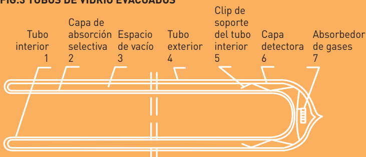
FIG.3 TUBOS DE VIDRIO EVACUADOS
